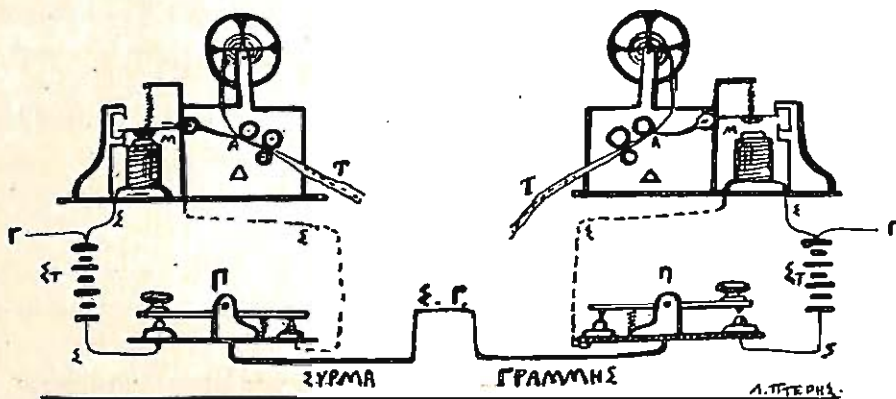
ΣΧΕΔΙΑΓΡΑΜΜΑ ΕΓΚΑΤΑΣΤΑΣΕΩΣ ΤΩΝ ΔΥΟ ΣΤΑΘΜΩΝ
